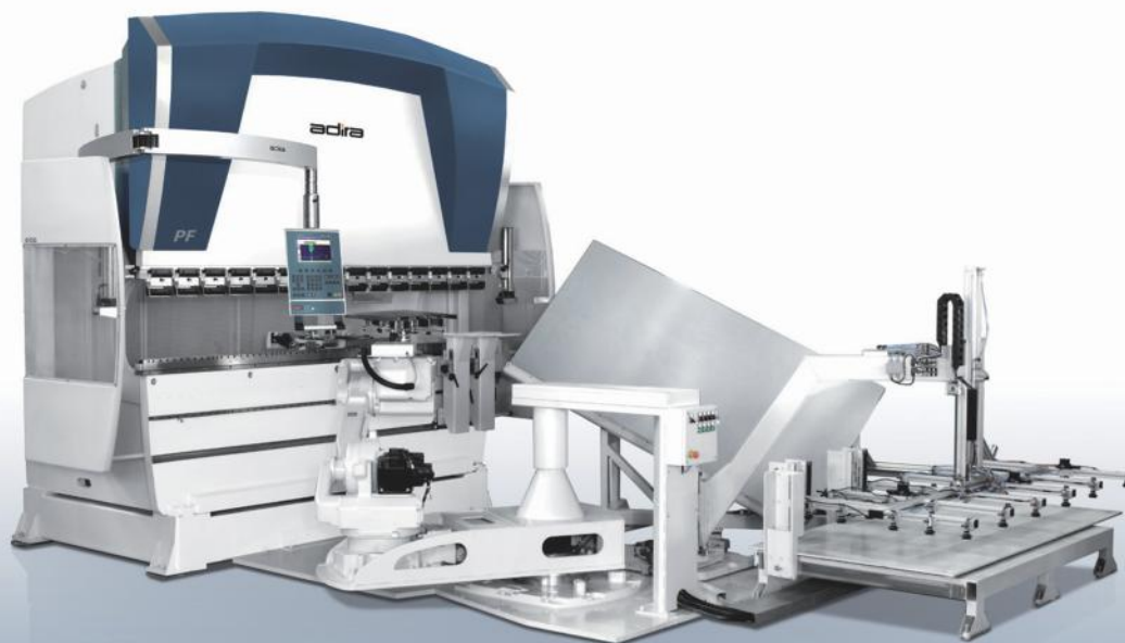
CELLULE ROBOTISEE DE PLIAGE
