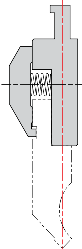
Attache LVD nez de 10, 15
