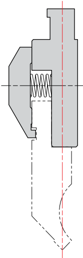
Attache COLLY nez de 13,5, 16
