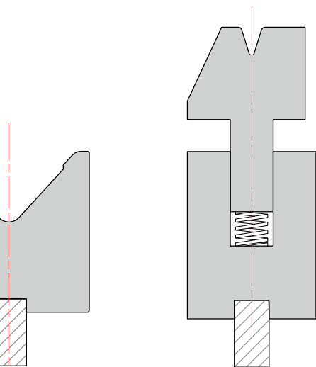
Rajout d'un talon pour adaptation sur Bystronic, Trumpf ou LVD
